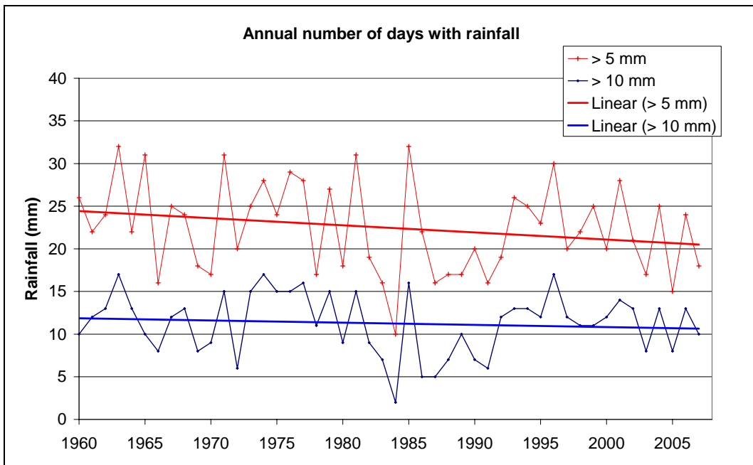
Rainfall trend Twee Rivieren
