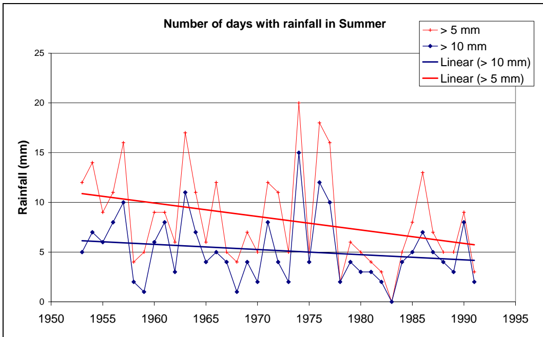
Rainfall trends Studtis (Baviaanskloof)
